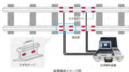
装置構成イメージ図
