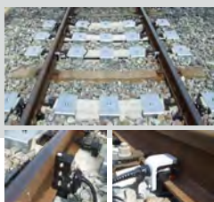
車輪検知センサ
